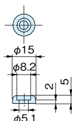
座金・スプリングW Washer・spring washer
