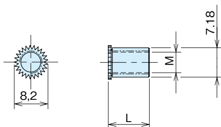
セルフクリンチングスペーサー
