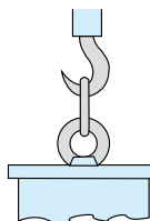
垂直つり
